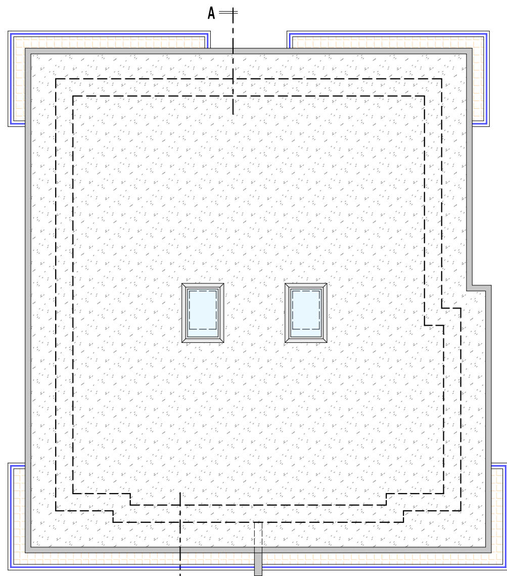
PIANTA DEL COPERTO
