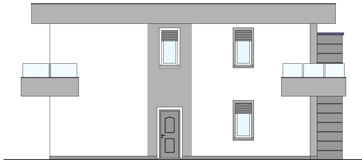
PROSPETTO LATO SINISTRO
