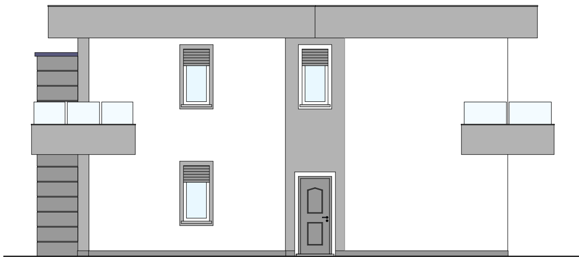
PROSPETTO LATO DESTRO
