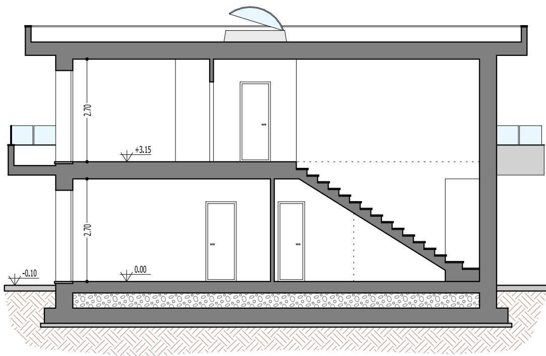
SEZIONE A-A
